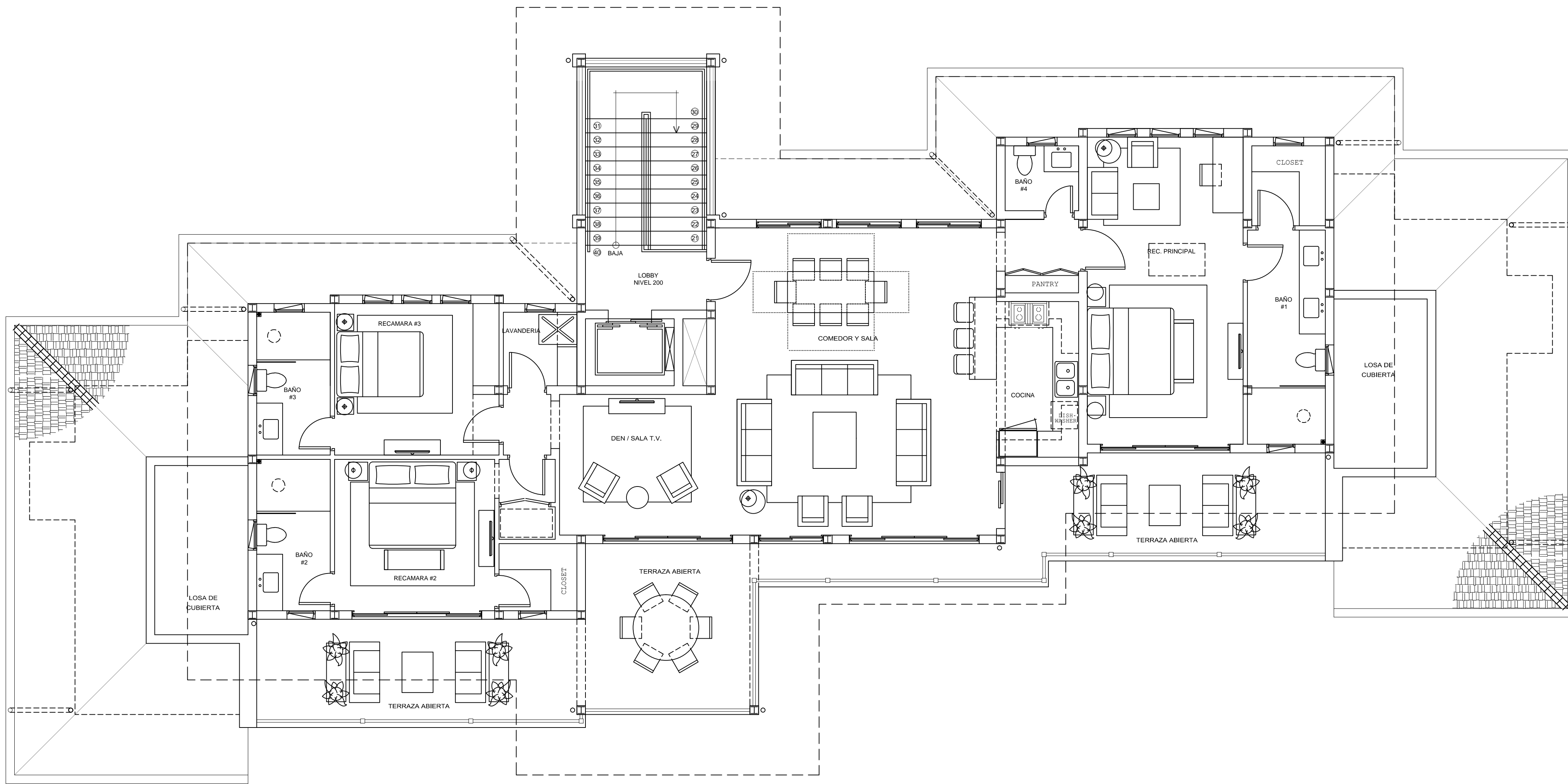
PLANTA NIVEL 200
