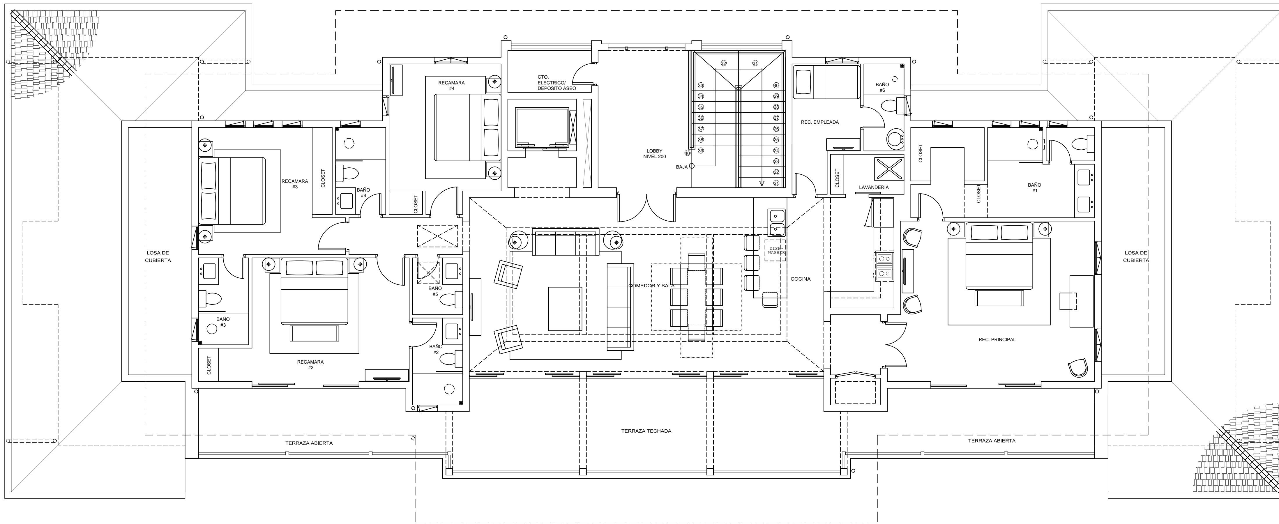
PLANTA NIVEL 200
