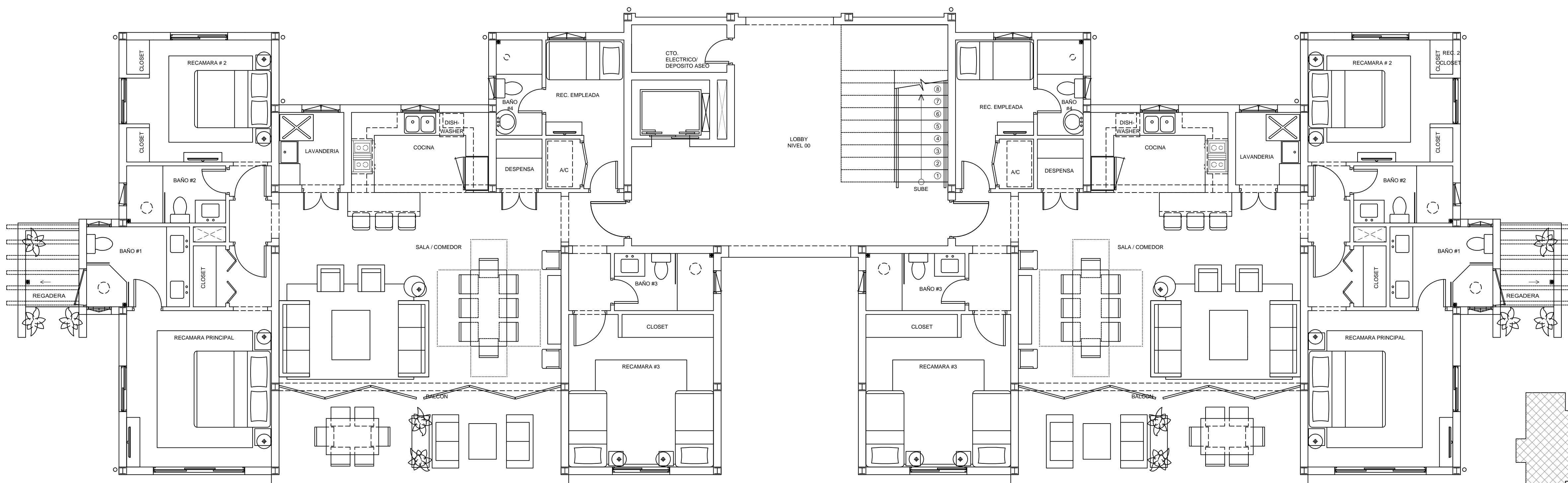
PLANTA NIVEL 000
