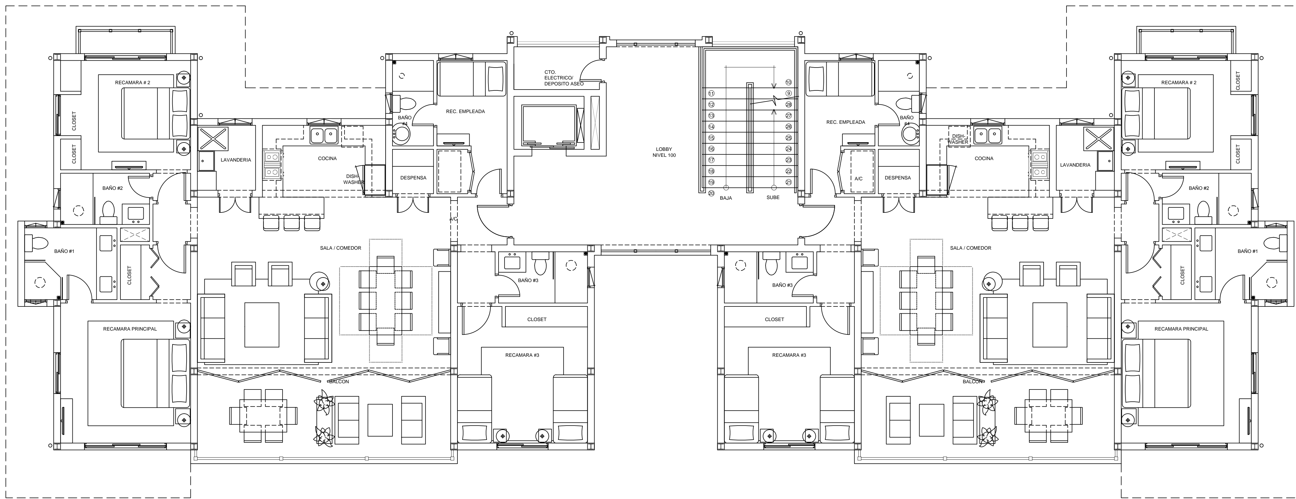
PLANTA NIVEL 100
