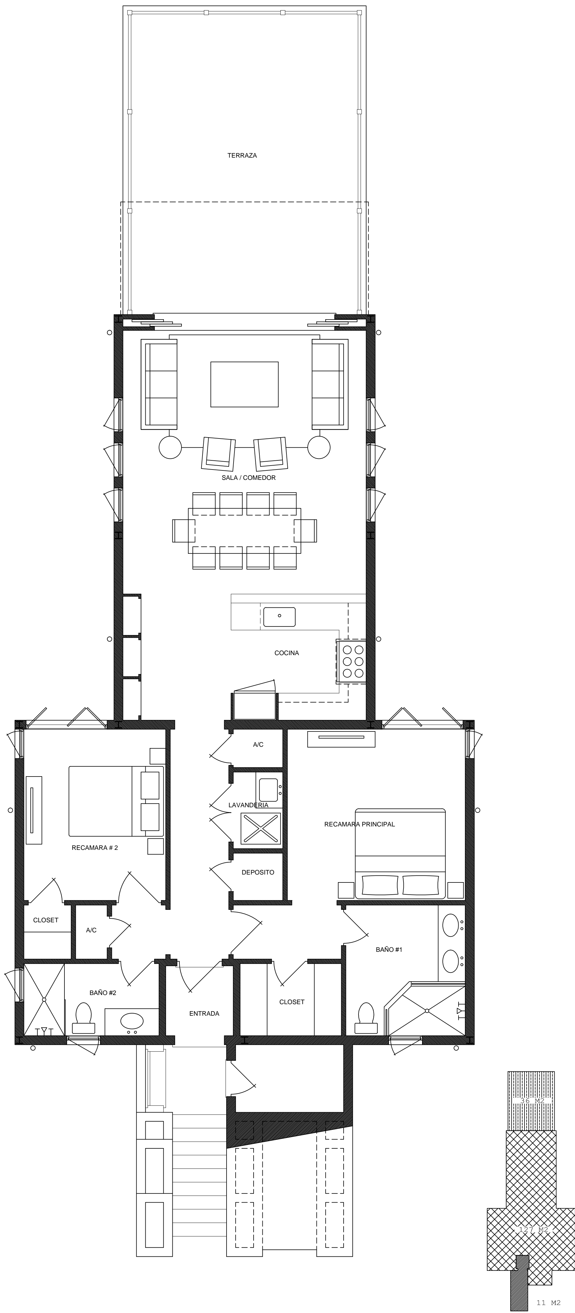
PLANTA NIVEL 000 - EDIFICIO E
