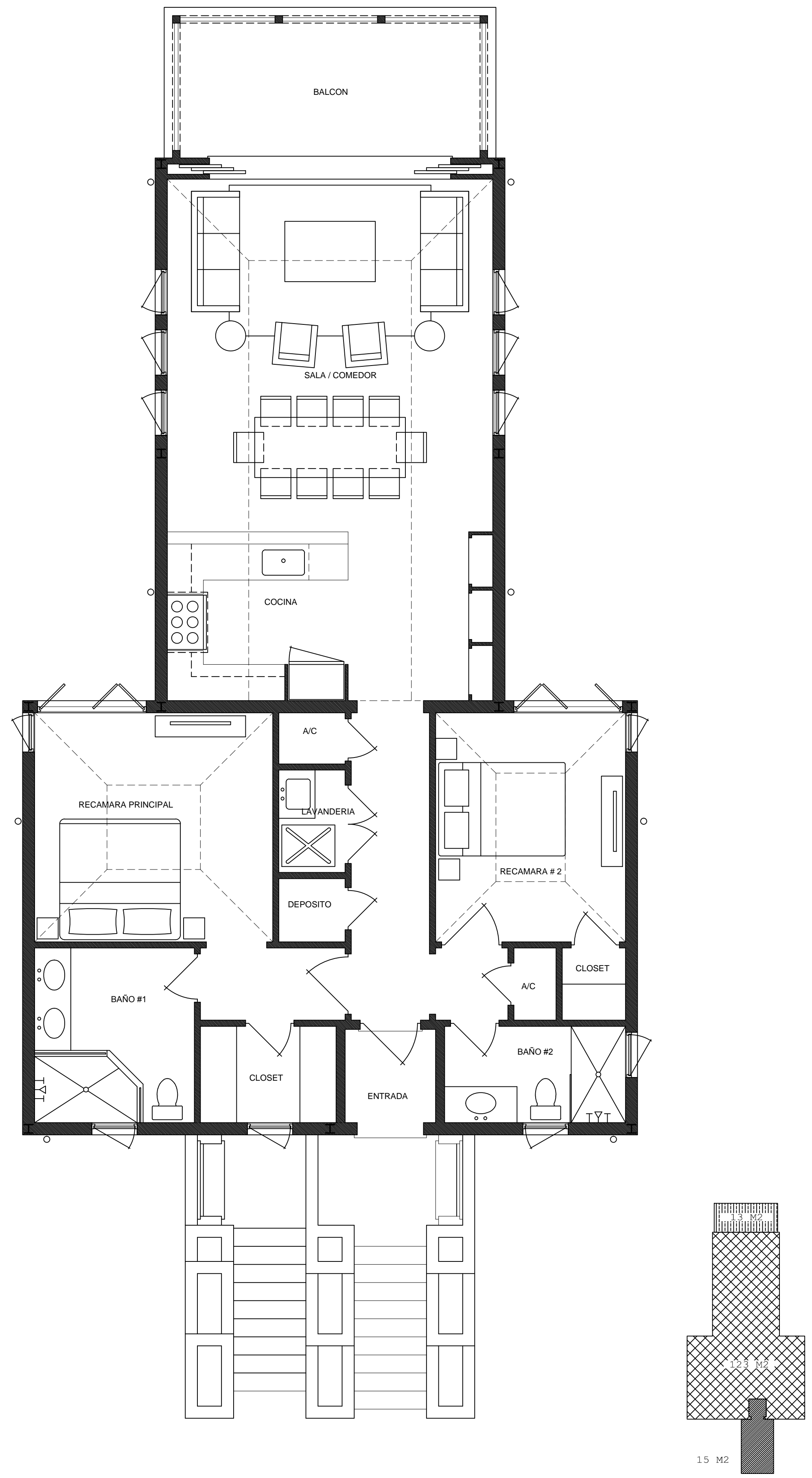
PLANTA NIVEL 100 - EDIFICIO E
